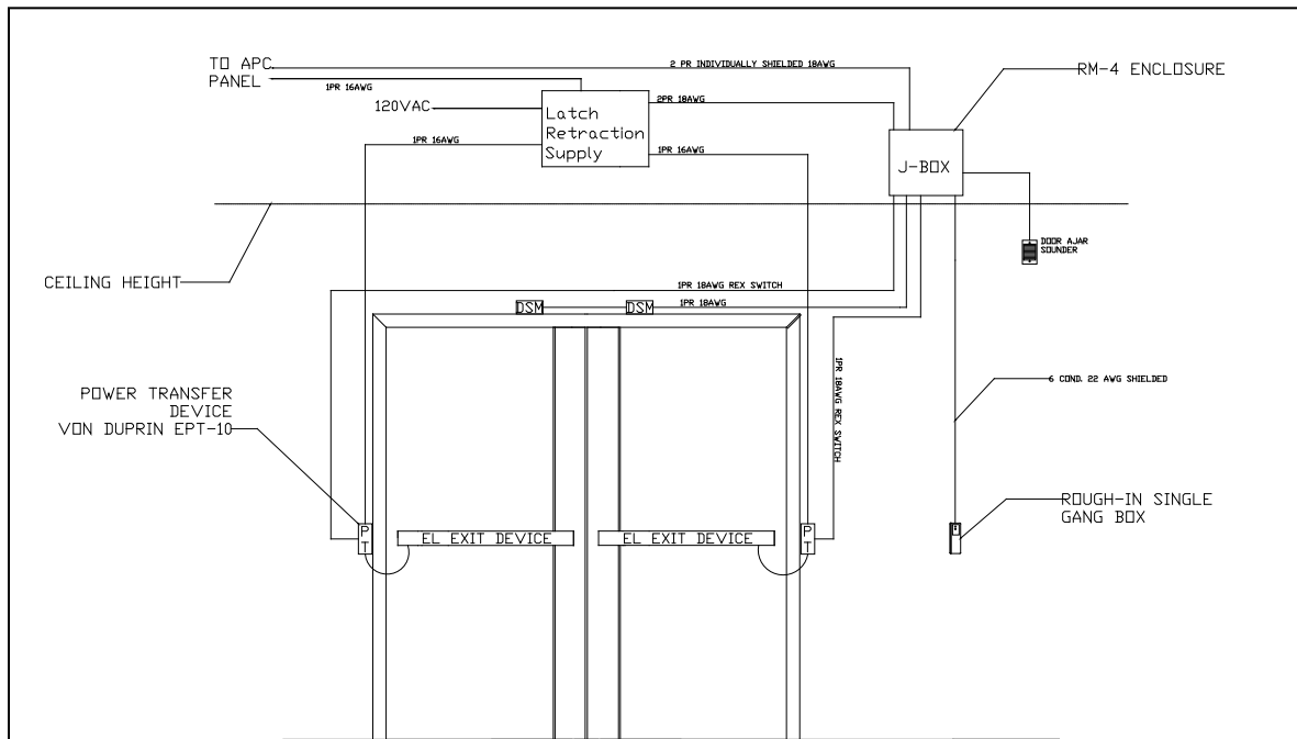
TYPE 2.35 CARD READER DOOR
